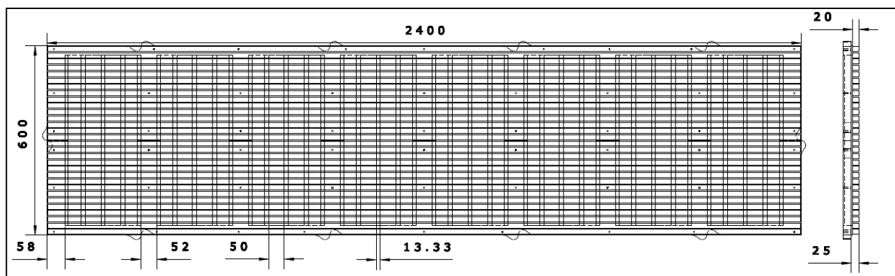
Vue en coupe d'un panneau 2,4 × 0,6 m
