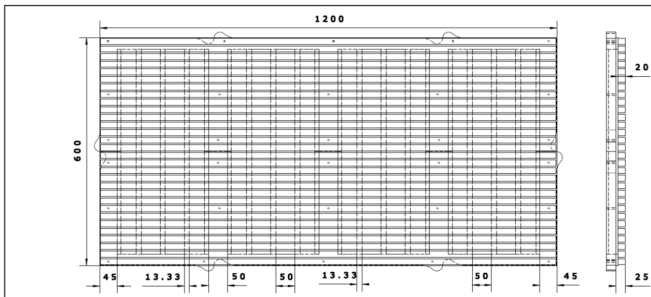
Vue en coupe d'un panneau 1,2 × 0,6 m
